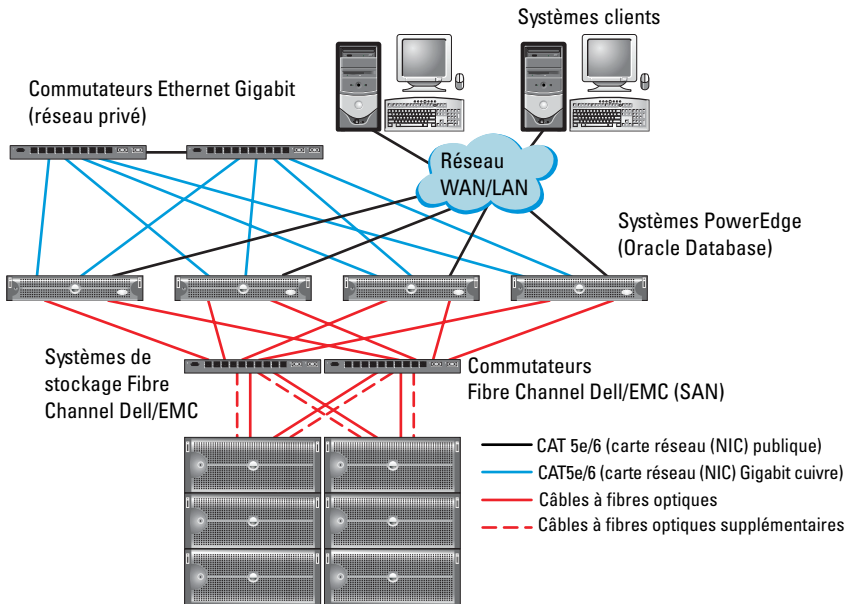
Figure 2-1. Connexions matérielles pour un cluster Fibre Channel
