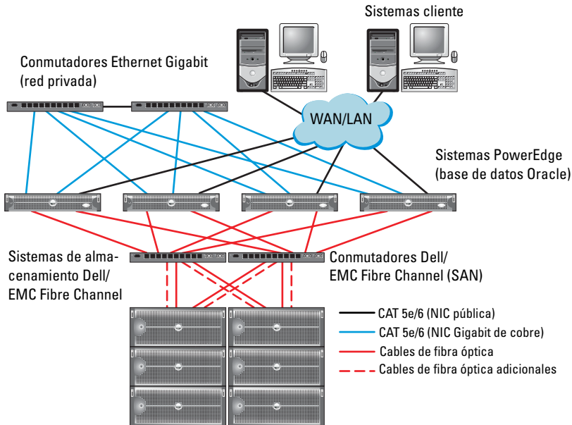
Ilustración 2-1. Conexiones de hardware para un clúster Fibre Channel
